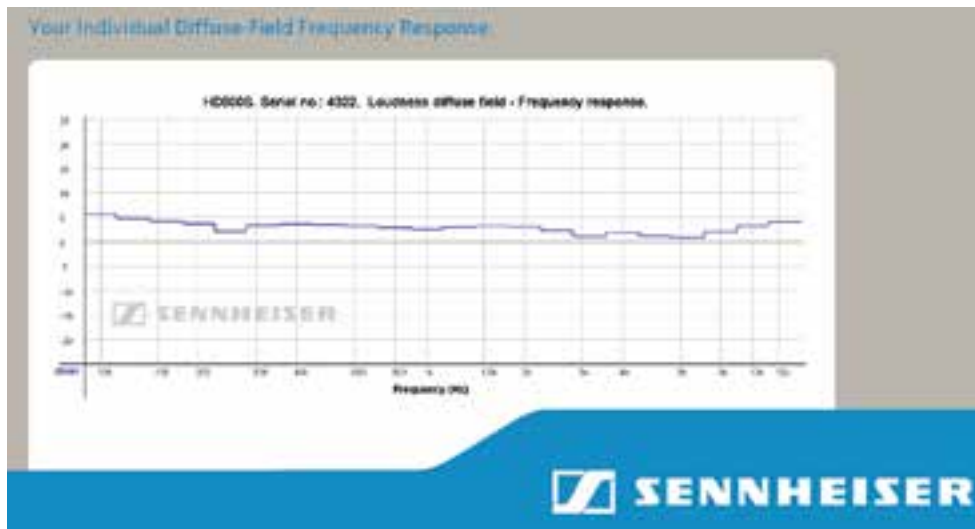
Courbe de réponse du casque HD 800 S de Sennheiser n°: 4322
